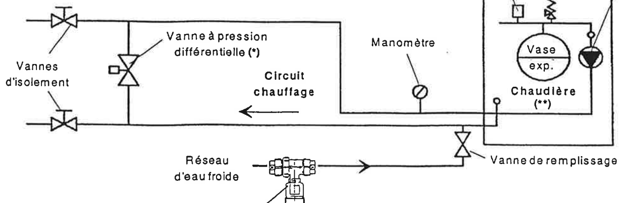
Raccordements hydrauliques et exemple d'installation
